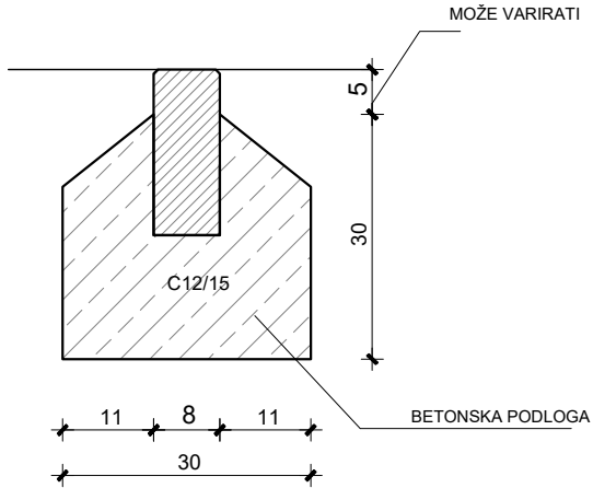
DETALJ UPUŠTENOG RUBNJAKA 8/20 cm
